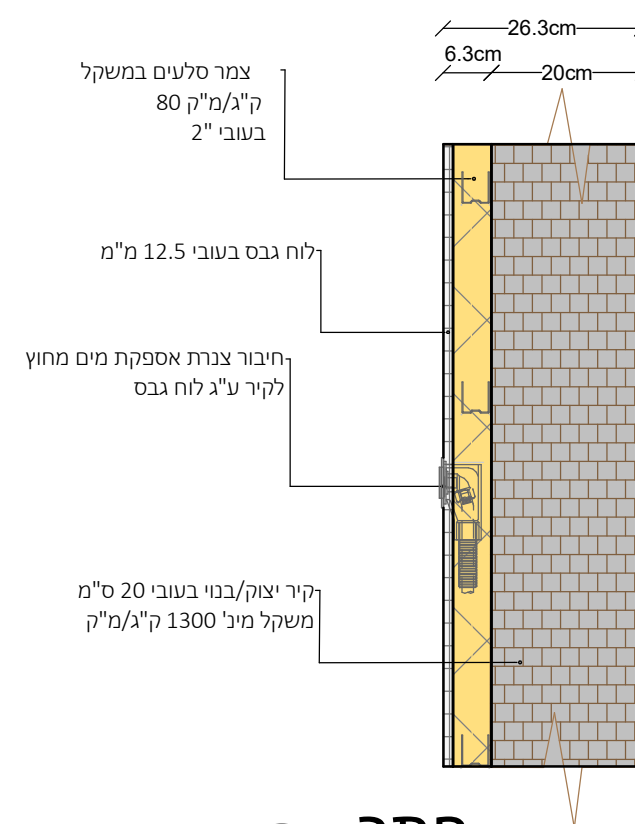
3 חתך 1 : 10
