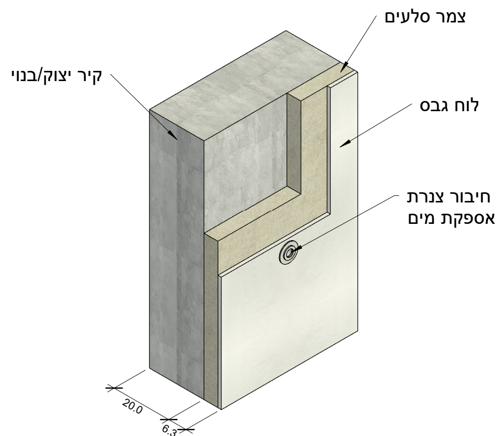
1 איזומטריה
